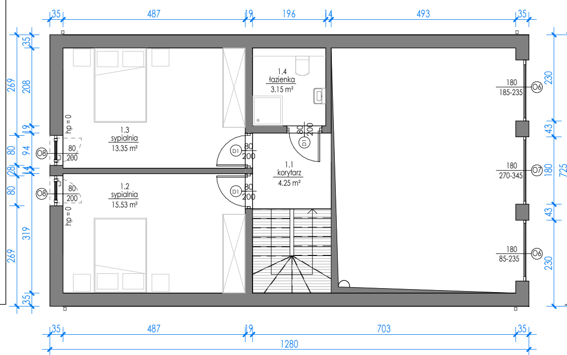
RZUT PODDASZA
