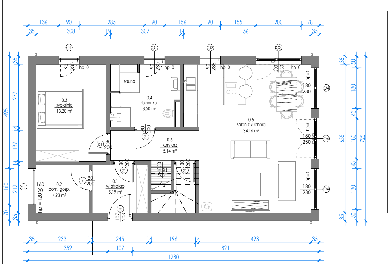
RZUT PARTERU
