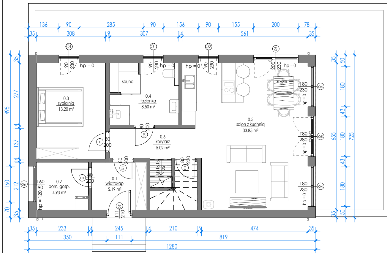
RZUT PARTERU
