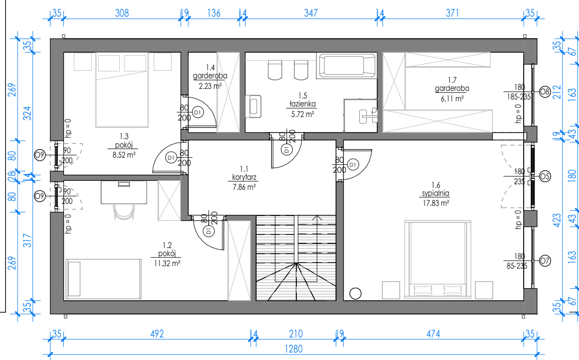
RZUT PODDASZA
