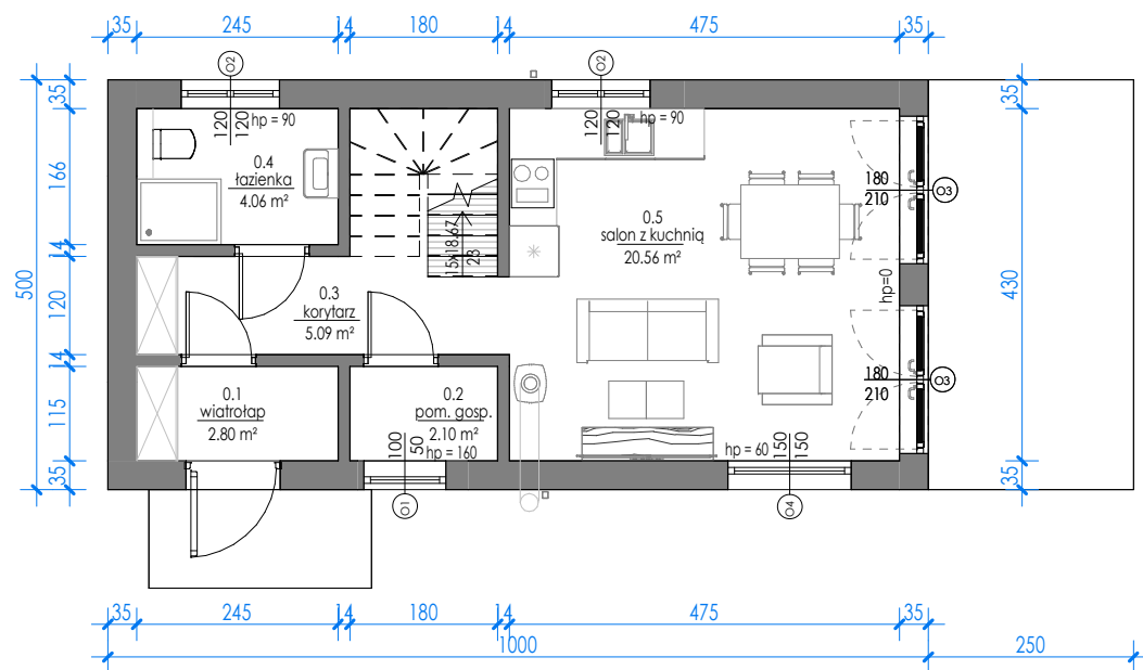
RZUT PARTERU
