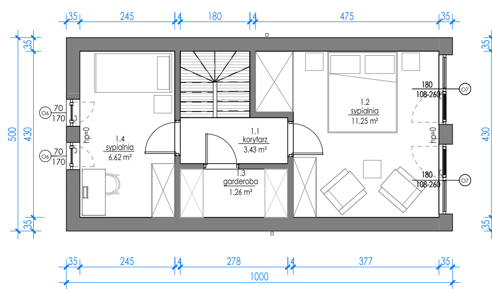
RZUT PODDASZA
