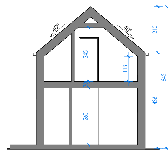
PRZEKRÓJ
