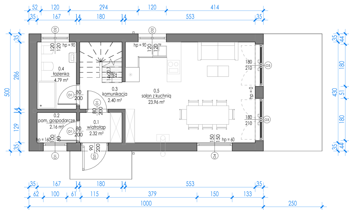
RZUT PARTERU
