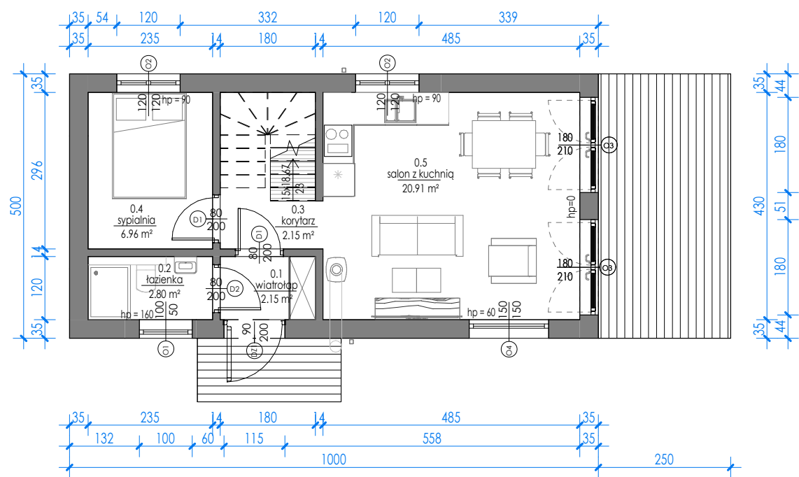
RZUT PARTERU
