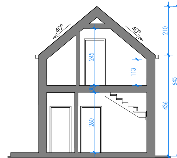
PRZEKRÓJ
