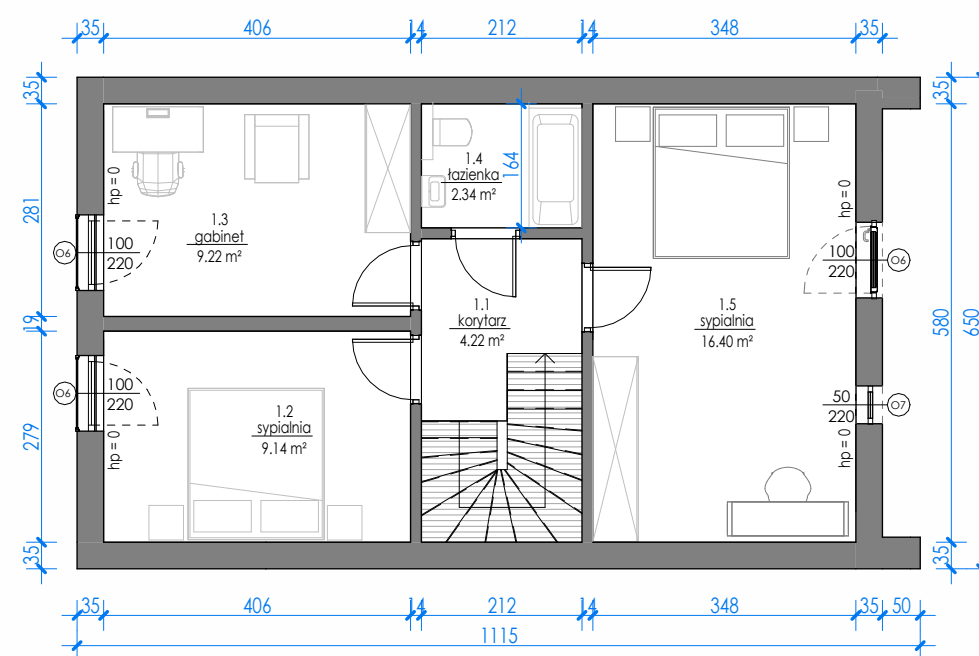
RZUT PODDASZA
