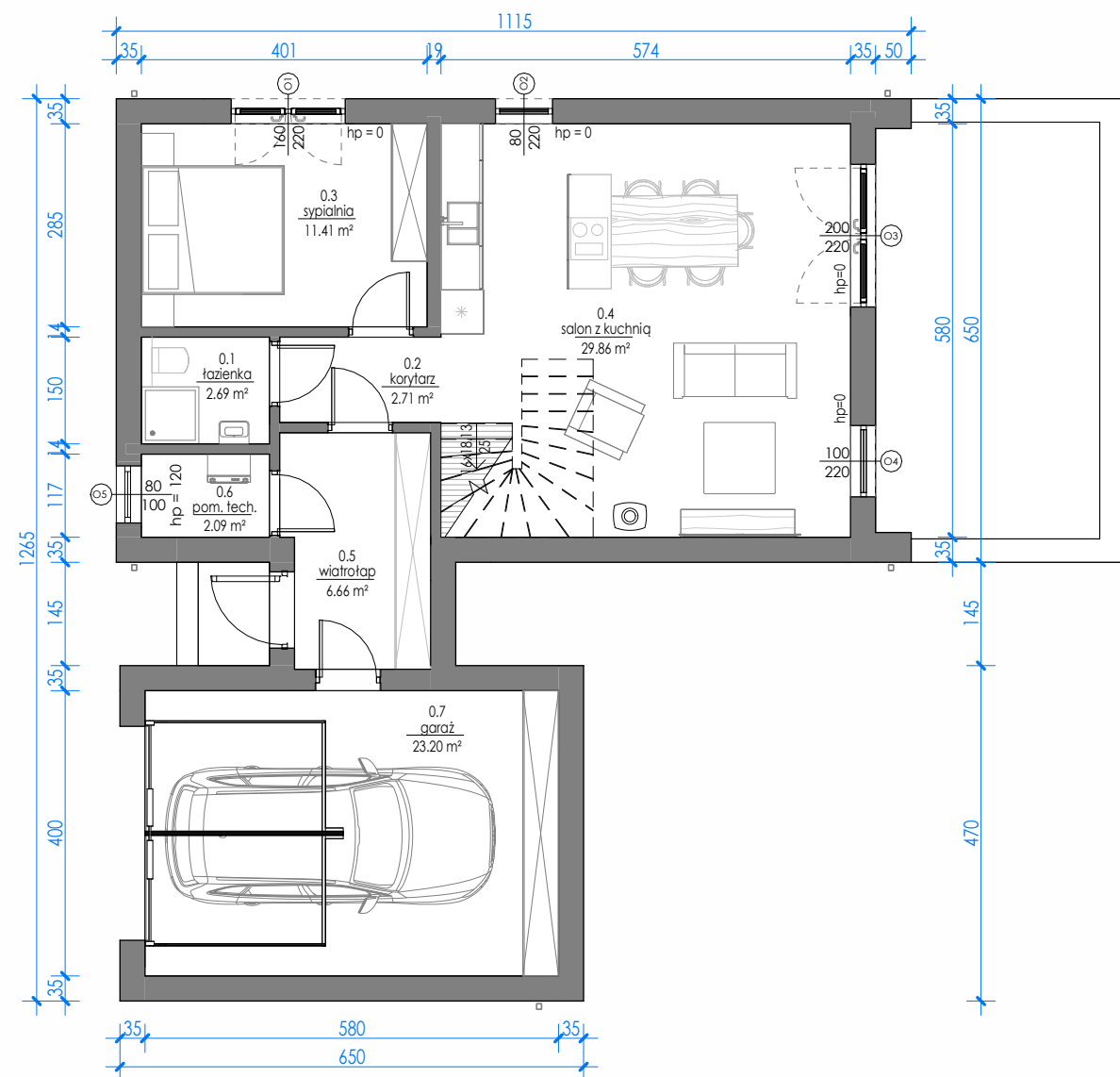
RZUT PARTERU
