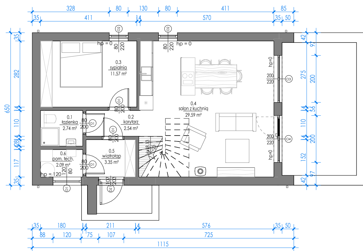
RZUT PARTERU
