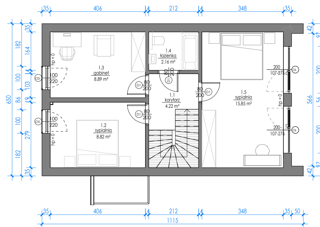
RZUT PODDASZA
