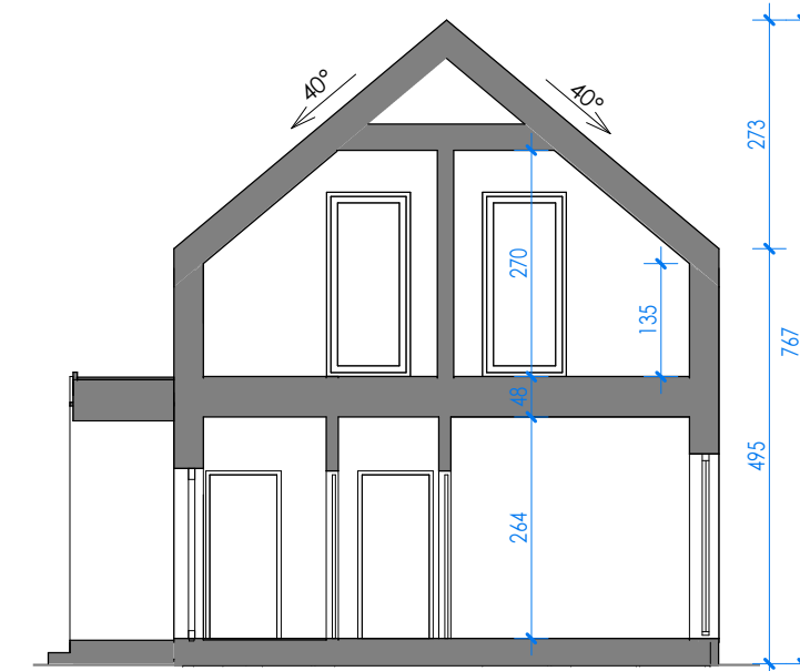
PRZEKRÓJ
