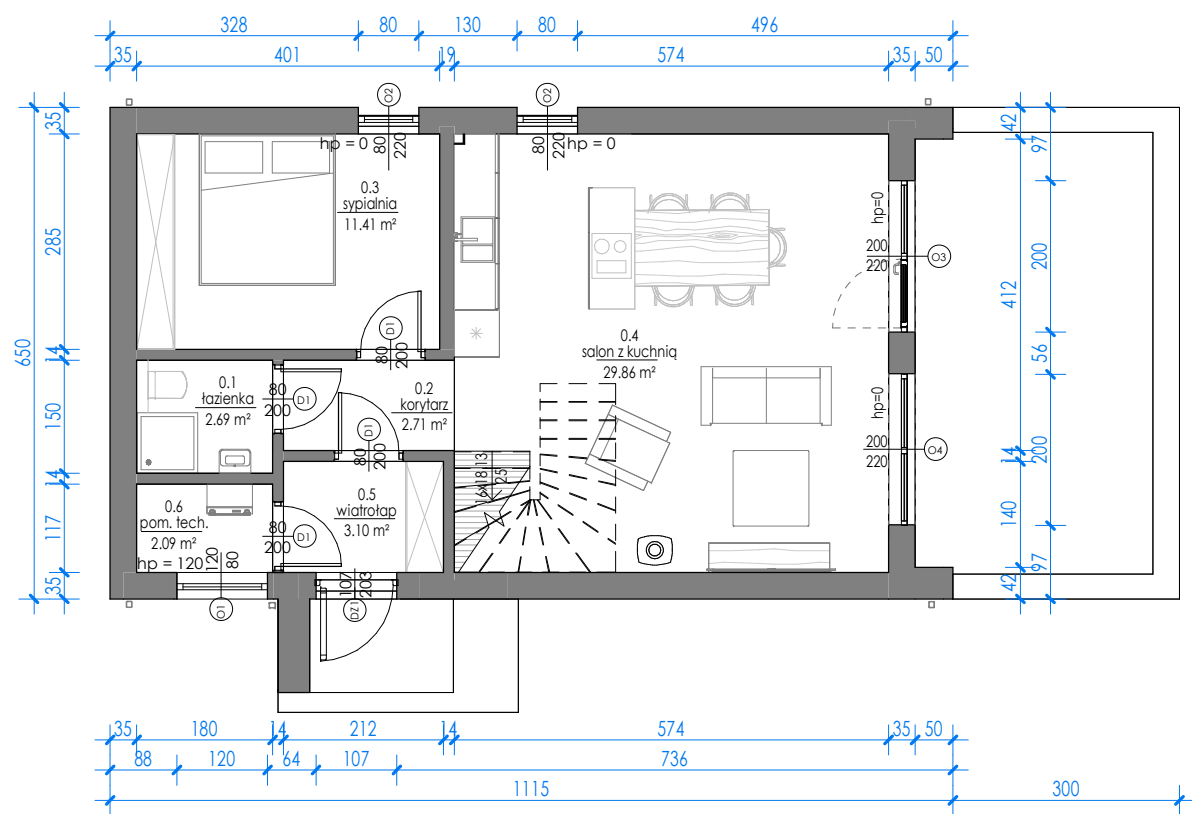
RZUT PARTERU
