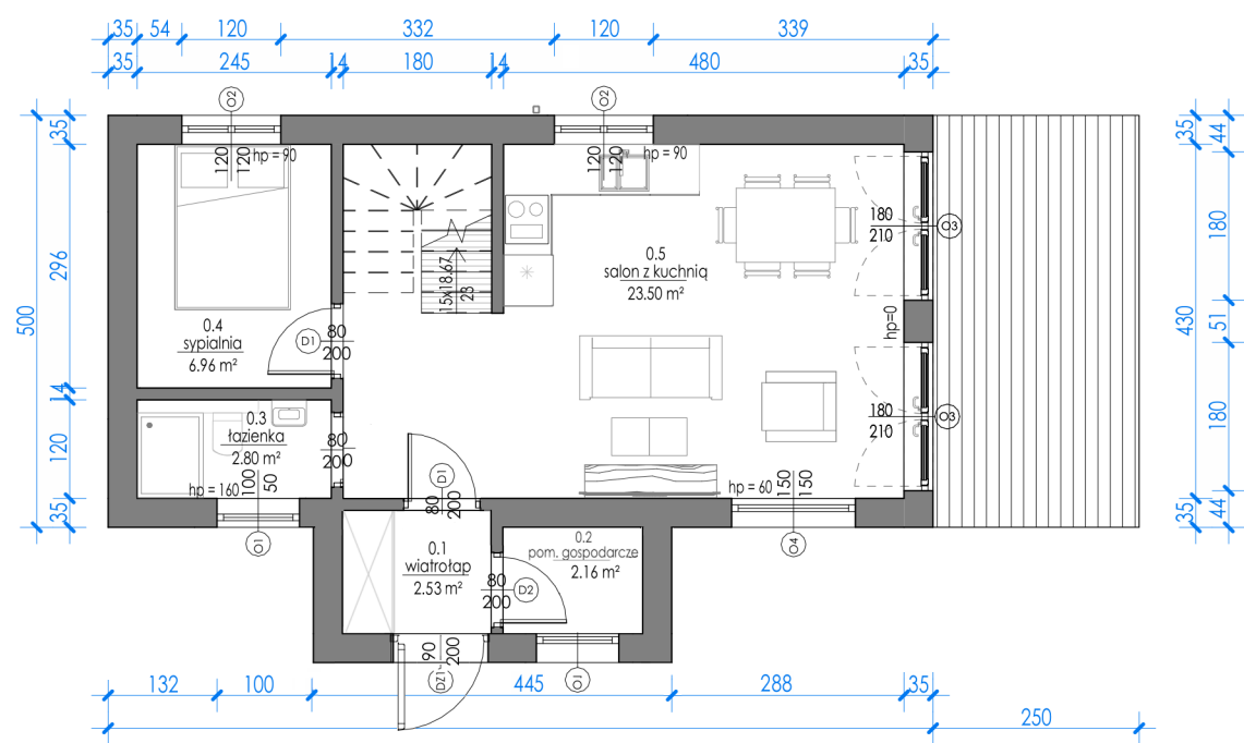
RZUT PARTERU
