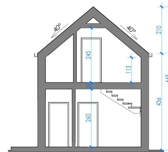
PRZEKRÓJ
