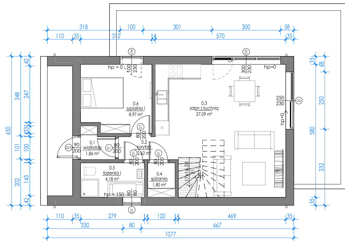
RZUT PARTERU
