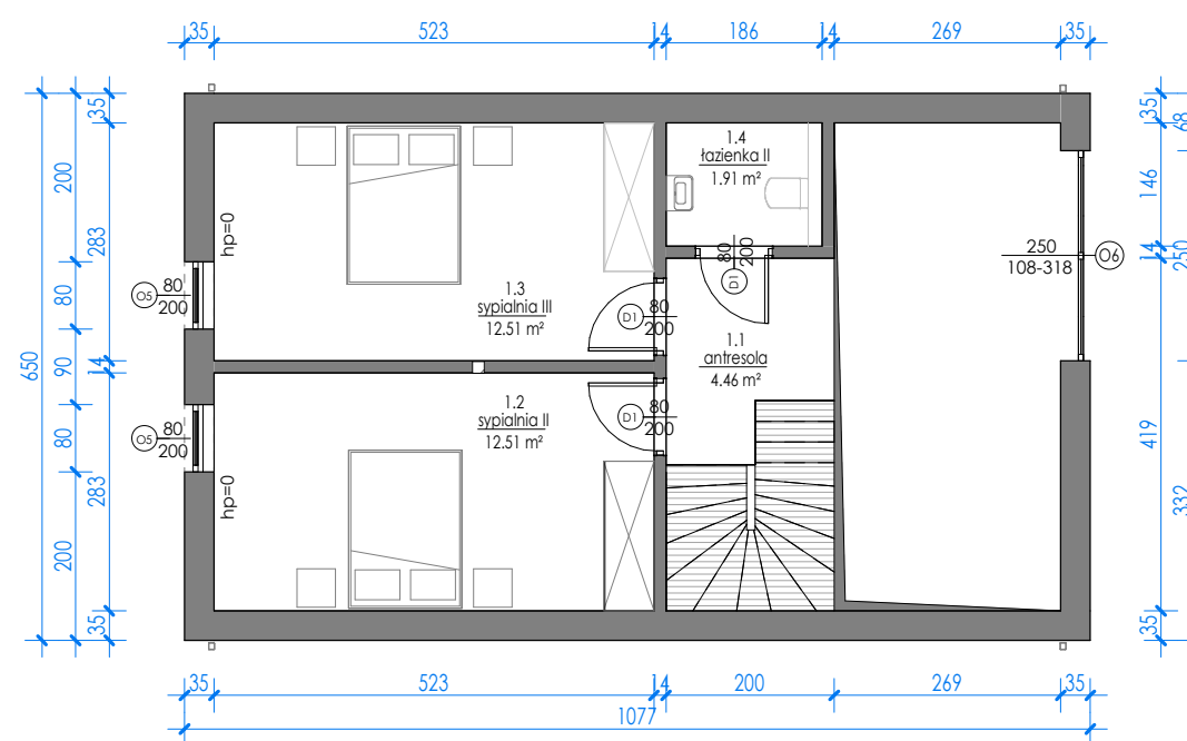
RZUT PODDASZA
