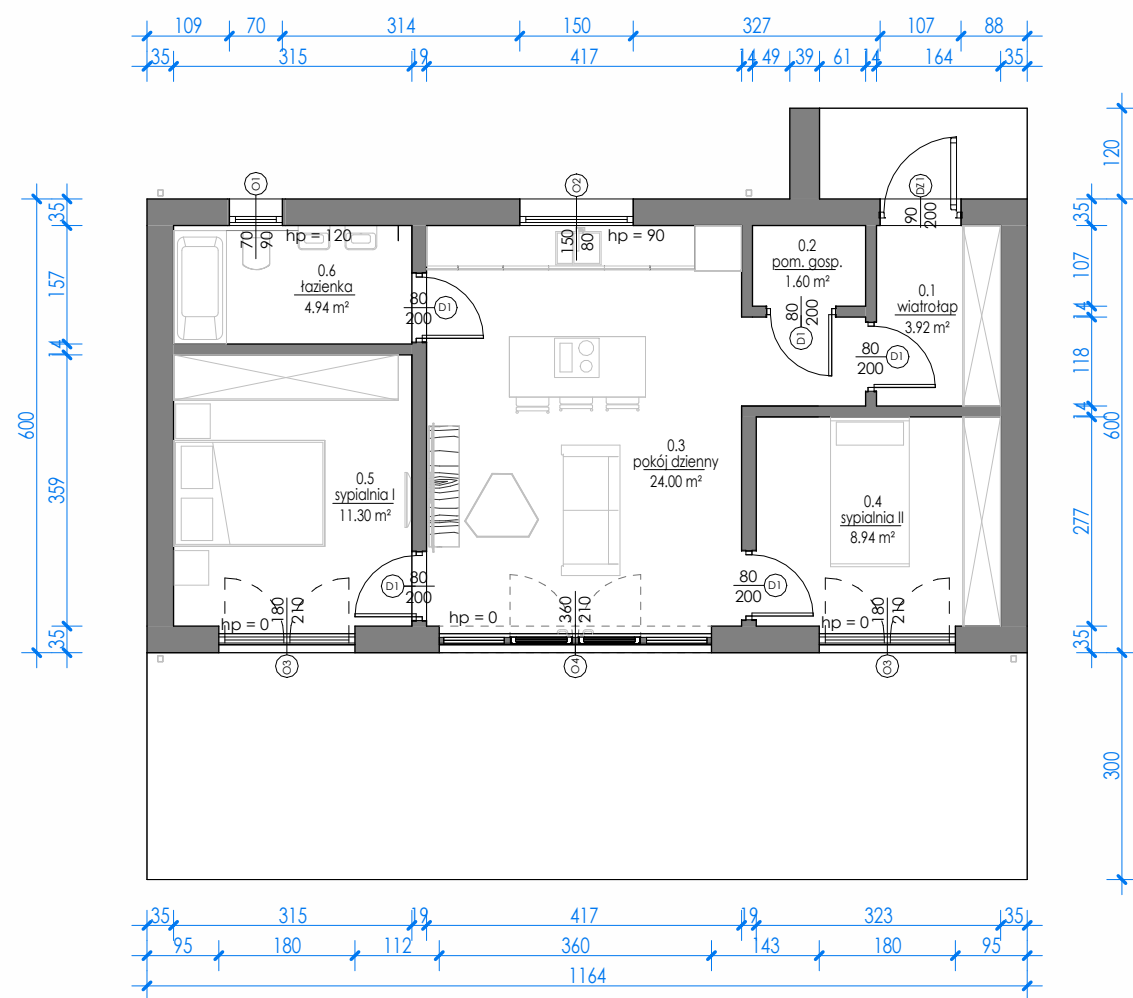
RZUT PARTERU
