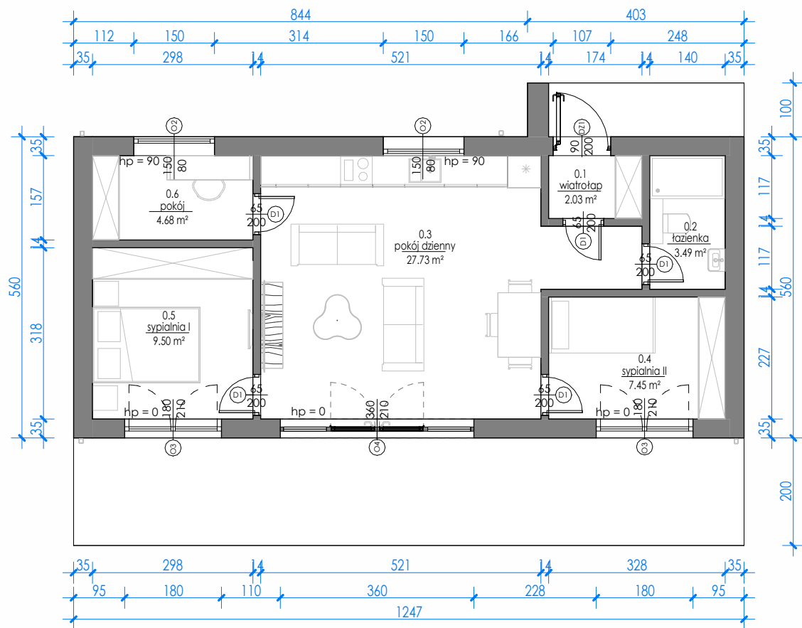
RZUT PARTERU
