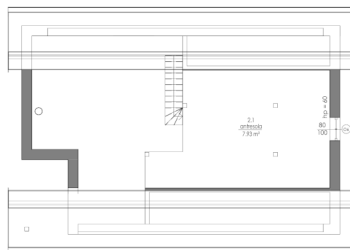
PODDASZE
