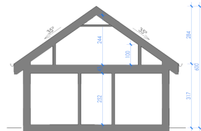
PRZECZÓJ
